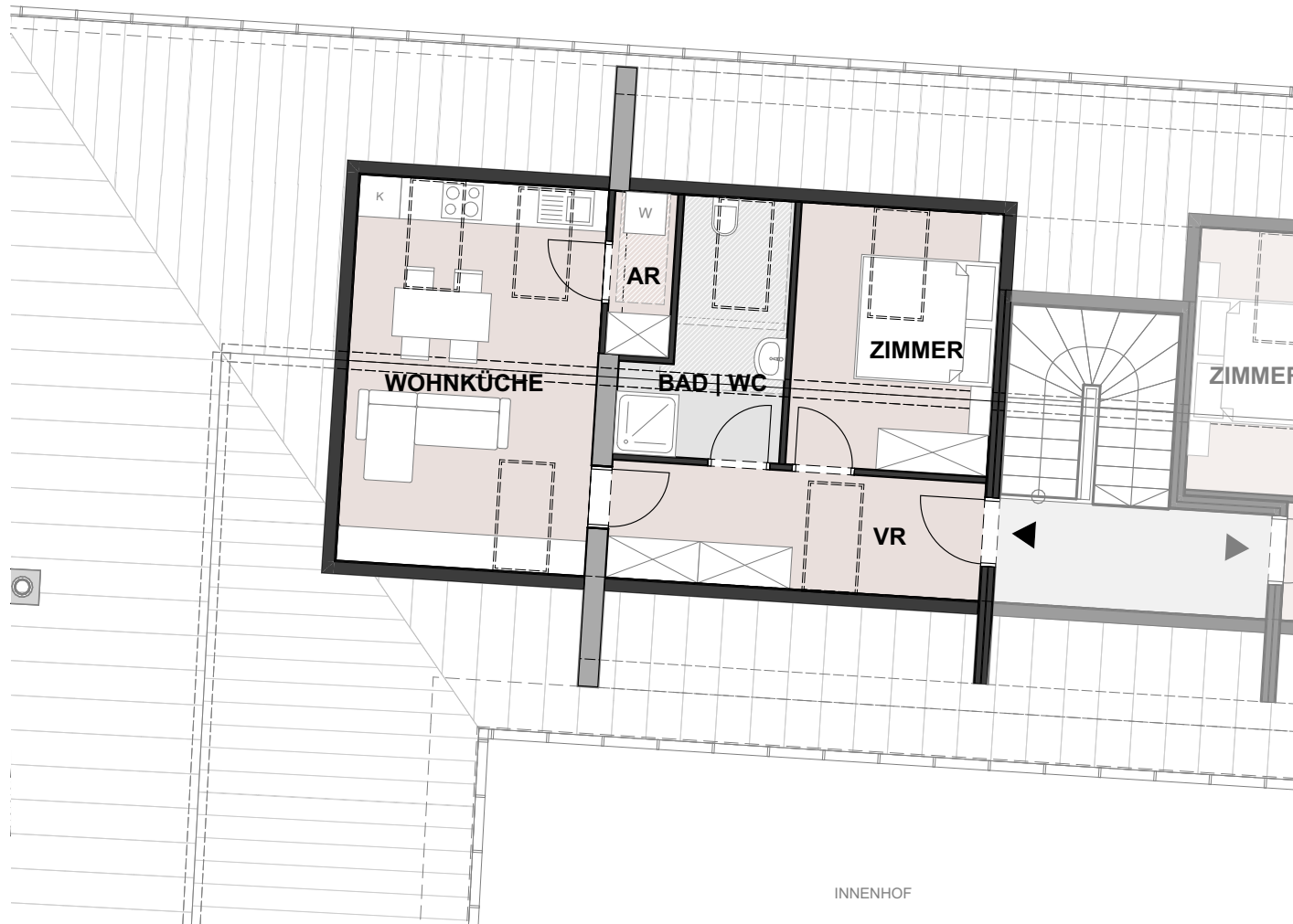
GRUNDRISS DACHGESCHOSS - TOP 16 M= 1:100
